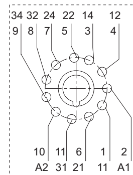
(顶视图)
