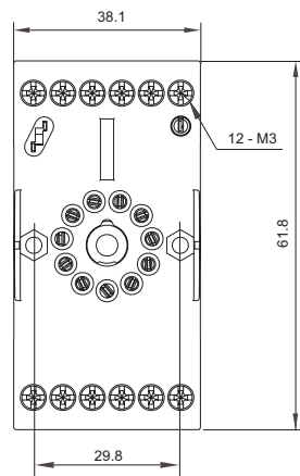
(顶视图)
