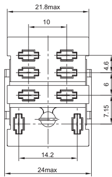
(顶视图)
