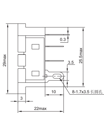
外形图
