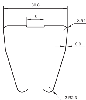
卡簧尺寸
