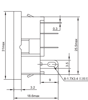
外形图
