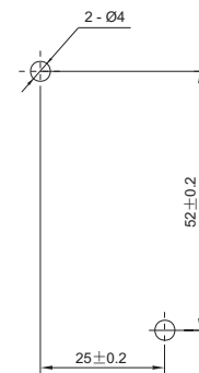
安装孔尺寸
