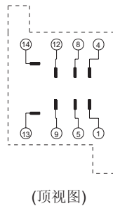
接线图
