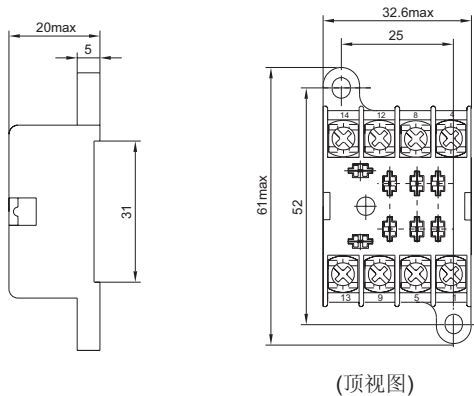
外形图
