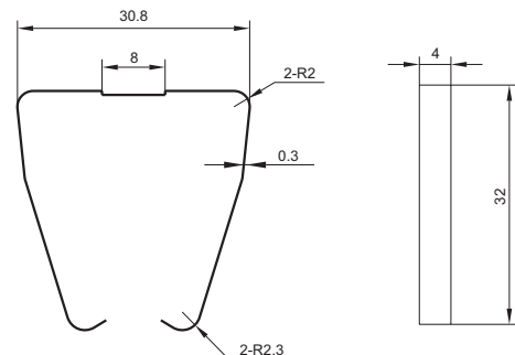
卡簧尺寸
