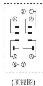
接线图
