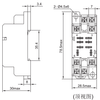
外形图
