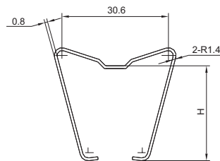
卡簧尺寸
