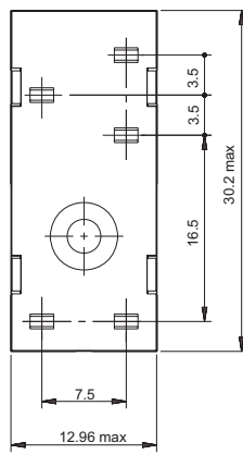
(顶视图)
