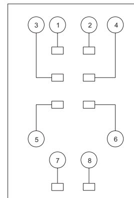
(顶视图)
