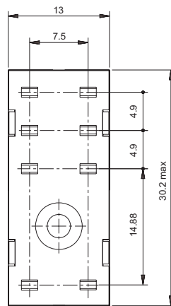
(顶视图)
