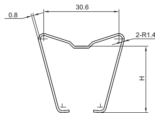
卡簧尺寸(-3 型)
