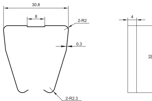
卡簧尺寸
