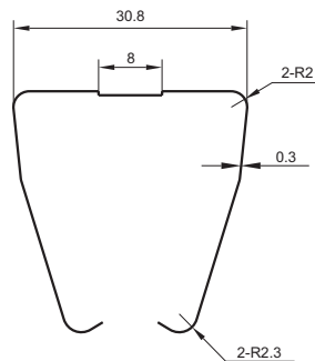
卡簧尺寸
