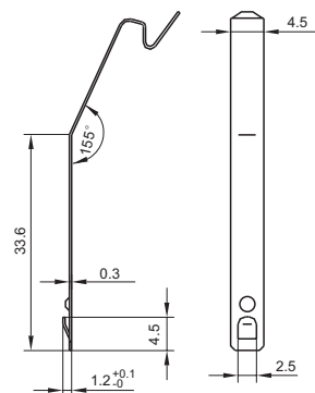
卡簧尺寸
