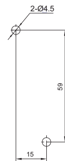
安装孔尺寸
