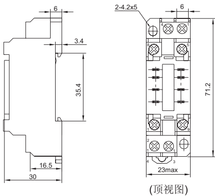
外形图
