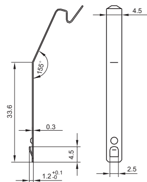
卡簧尺寸
