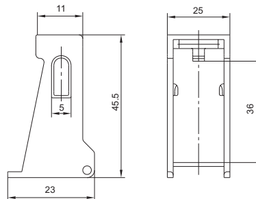
卡簧尺寸
