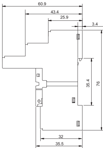
外形图
