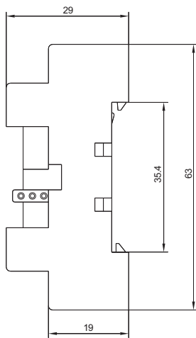
外形图
