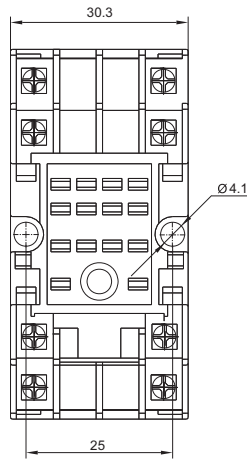
(顶视图)
