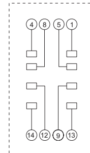
(顶视图)
