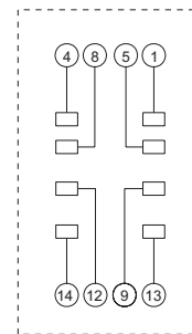
(顶视图)
