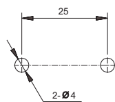
安装孔尺寸
