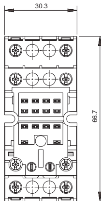
(顶视图)
