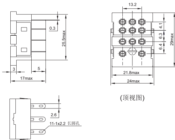
外形图
