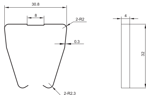
卡簧尺寸
