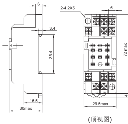
外形图
