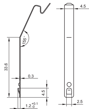
卡簧尺寸
