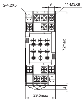
(顶视图)
