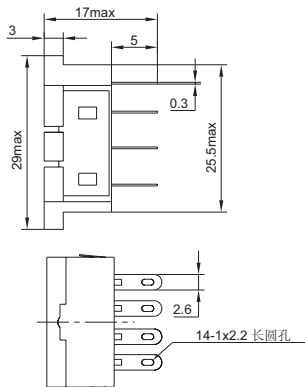
外形图
