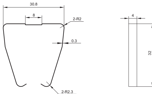
卡簧尺寸
