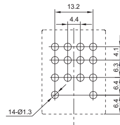
安装孔尺寸
