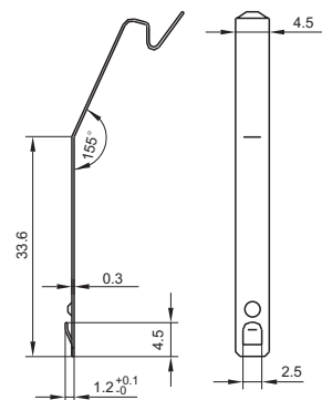
卡簧尺寸
