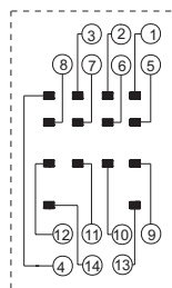
(顶视图)
