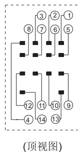
接线图
