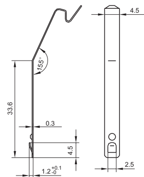
卡簧尺寸
