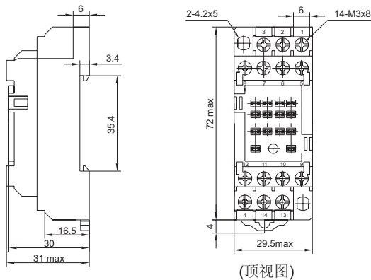
外形图
