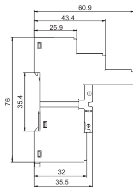
外形图
