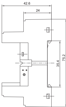
外形图
