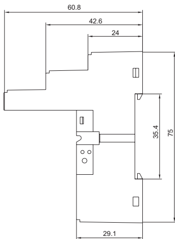
外形图
