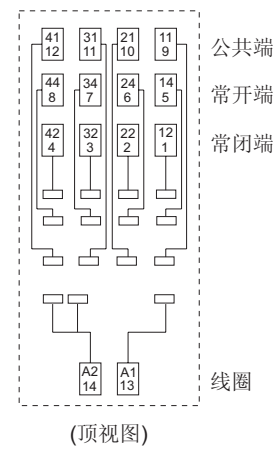
接线图
