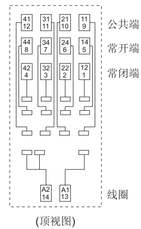
接线图
