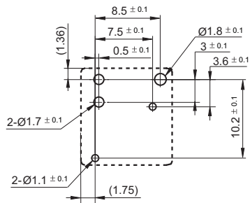
单继电器
