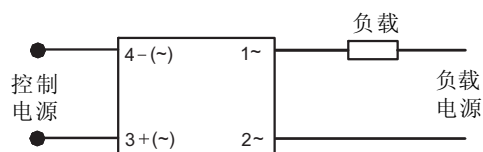
接线图
