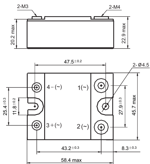
外形图
