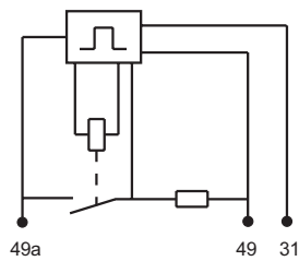
接线图
