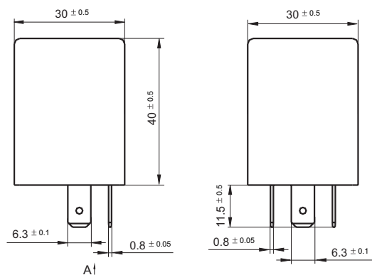
外形图
