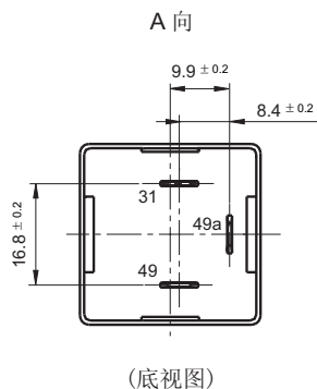
引出脚位图
