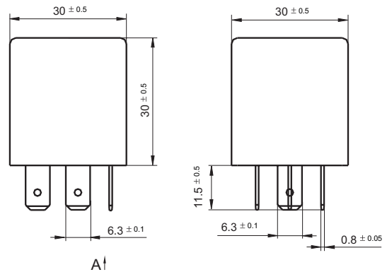
外形图
