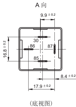
引出脚位图
