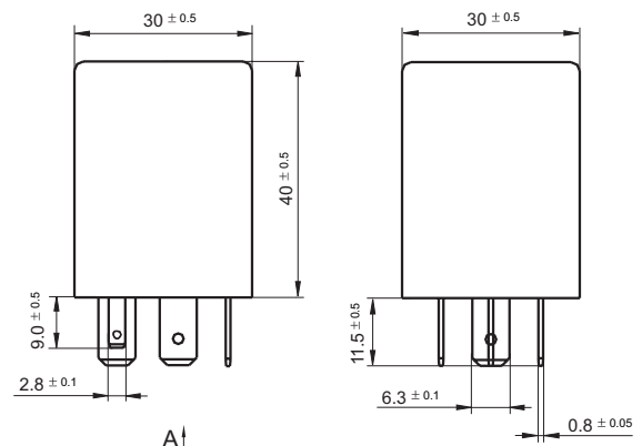
外形图
