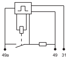
接线图
