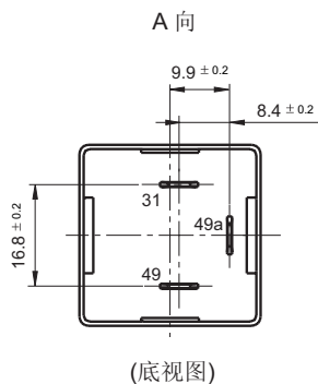
引出脚位图
