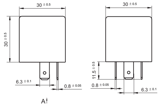
外形图
