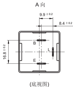
引出脚位图
